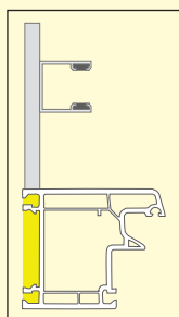
Vodiaca lišta NB 28 - pripevnenie na omietku ostena otvoru
