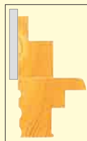
Drevené okno pripravené na montáž vodiacej lišty NB 28
